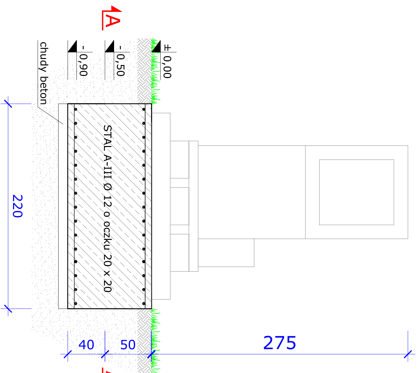
PRZEKRÓJ A-A
